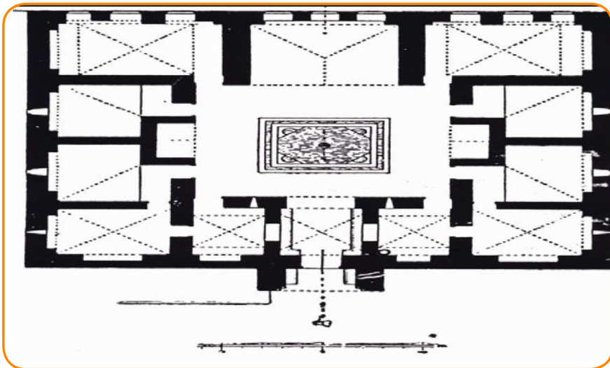
نەخشەى بناغەى نەخۆشخانەى تەيمورى لە ديمەشق
